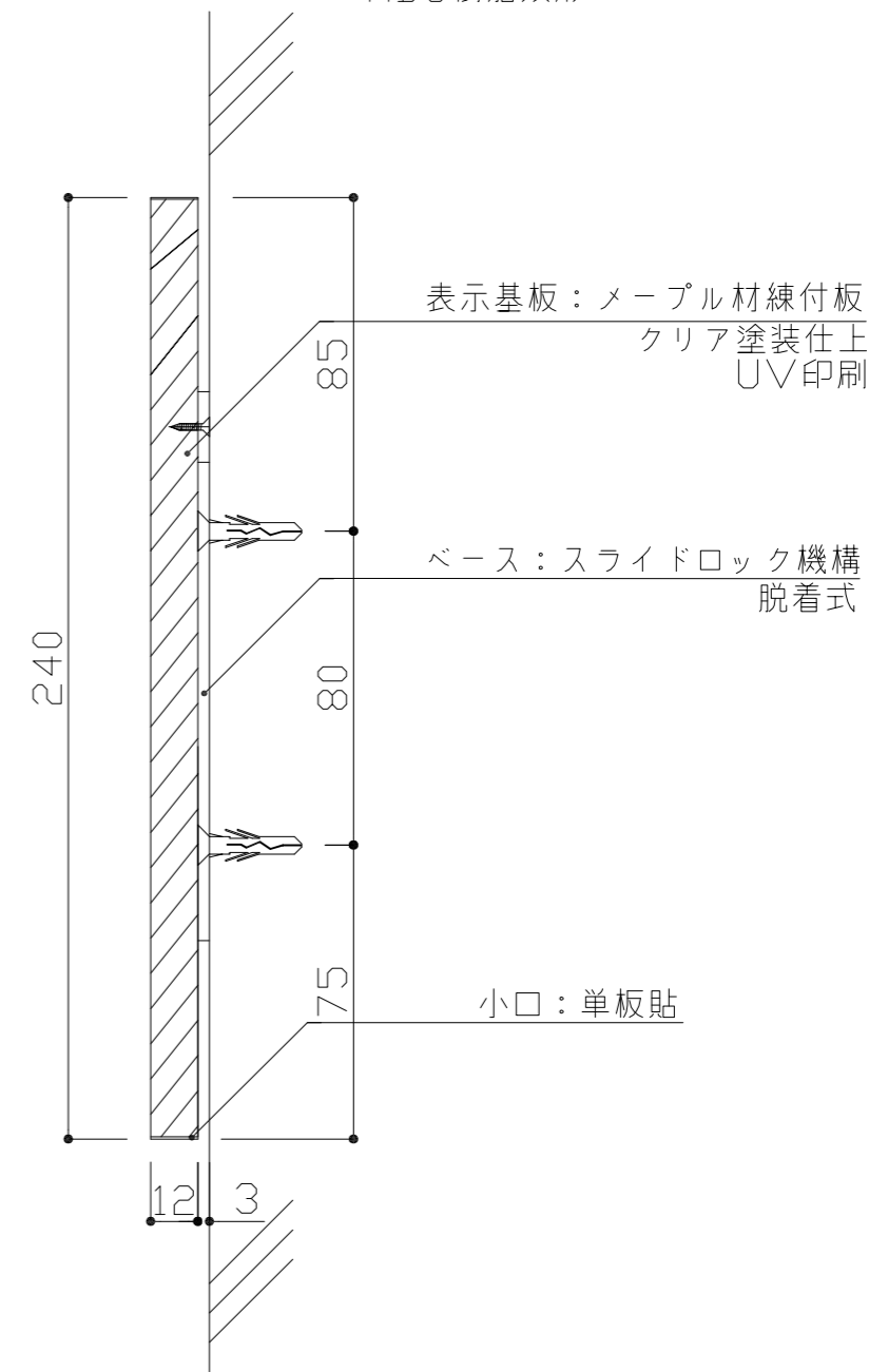
※スライドロック機構 脱着式 (ABS樹脂成形)
